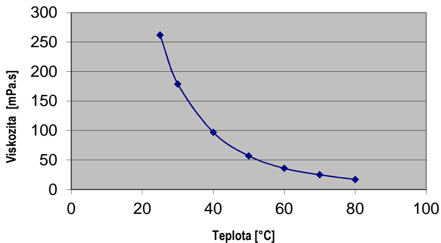
Závislosť viskozity NH 91 LV od teploty
